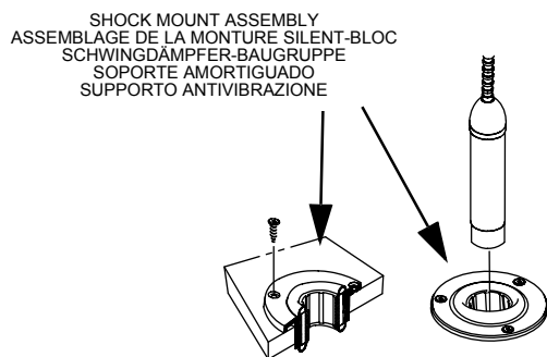
SHOCK MOUNT INSTALLATION • INSTALLATION DE LA MONTURE SILENT-BLOC • INSTALLATION DES SCHWINGDÄMPFERS • INSTALACION DEL SOPORTE AMORTIGUADO • INSTALLAZIONE DEL SUPPORTO ANTIVIBRAZIONE
