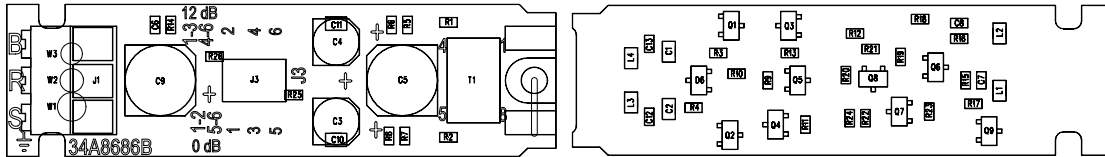
MX412/MX418 CIRCUIT BOARD LEGEND • LÉGENDE DU CIRCUIT IMPRIMÉ MX412/MX418 • BESCHRIFTUNG DER MX412/MX418 LETTERPLATTE • LEYENDA DE CIRCUITOS DE MX412/MX418 • LEGENDA DELLA SCHEDA DI CIRCUITI DEI MODELLI MX412/MX418
