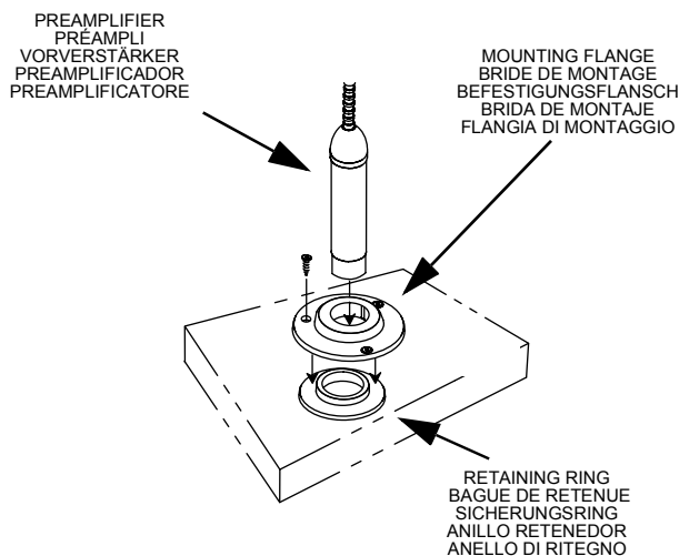
MOUNTING FLANGE INSTALLATION • INSTALLATION DE LA BRIDE DE MONTAGE • INSTALLATION DES BEFESTIGUNGSFLANSCHES • INSTALACION DE BRIDA DE MONTAJE • INSTALLAZIONE DELLA FLANGIA DI MONTAGGIO
