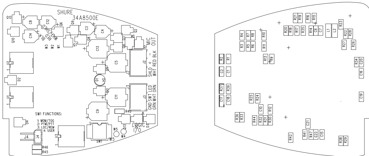
MX392/MX393 CIRCUIT BOARD LEGEND LÉGENDE DU CIRCUIT IMPRIMÉ MX392/MX393 BESCHRIFTUNG DER MX392/MX393 LEITERPLATTE LEYENDA DE TARJETA DE CIRCUITOS DE MX392/MX393 LEGENDA DELLA SCHEDA DI CIRCUITI DEI MODELLI MX392/MX393
